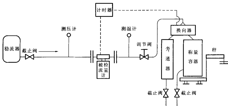
图 1 质量法检定流程图
