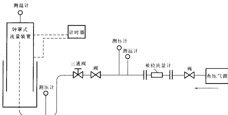
图5 钟罩式流量装置检定流程图
