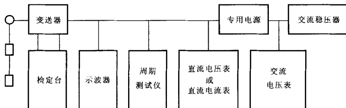
静态检定流程框图
