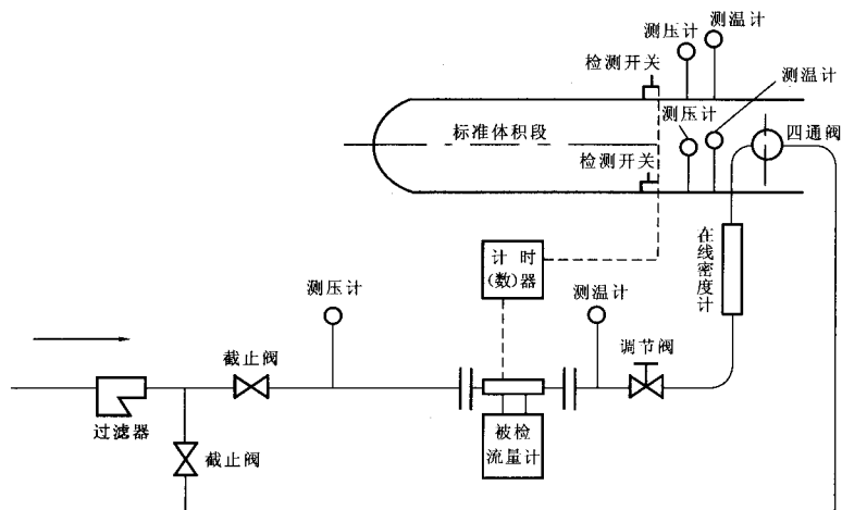
图3 体积管法检定流程图
