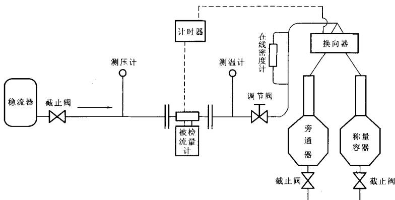
图 2 容积法检定流程图
