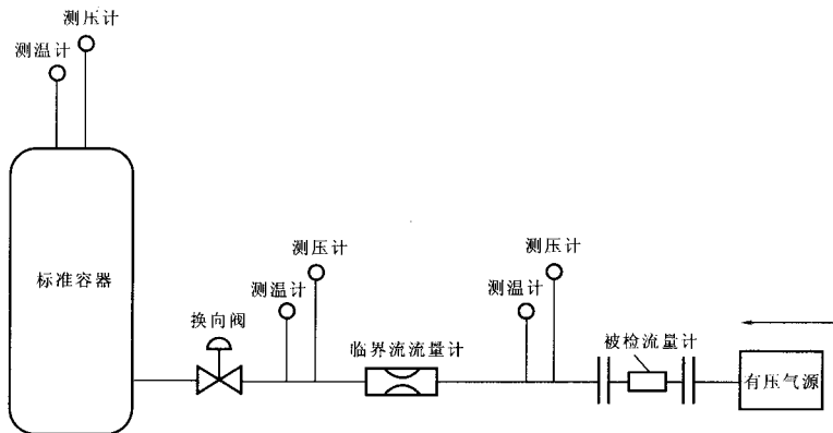
图6 临界流流量计检定流程图
