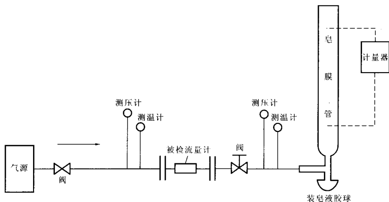
图4 皂膜式流量装置检定流程图
